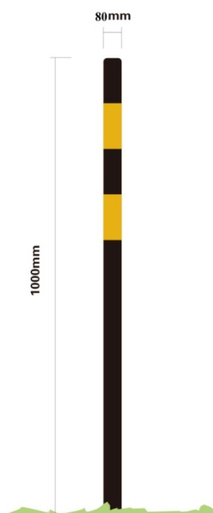
图 A.4 地下水监测井警示柱图示及尺寸
